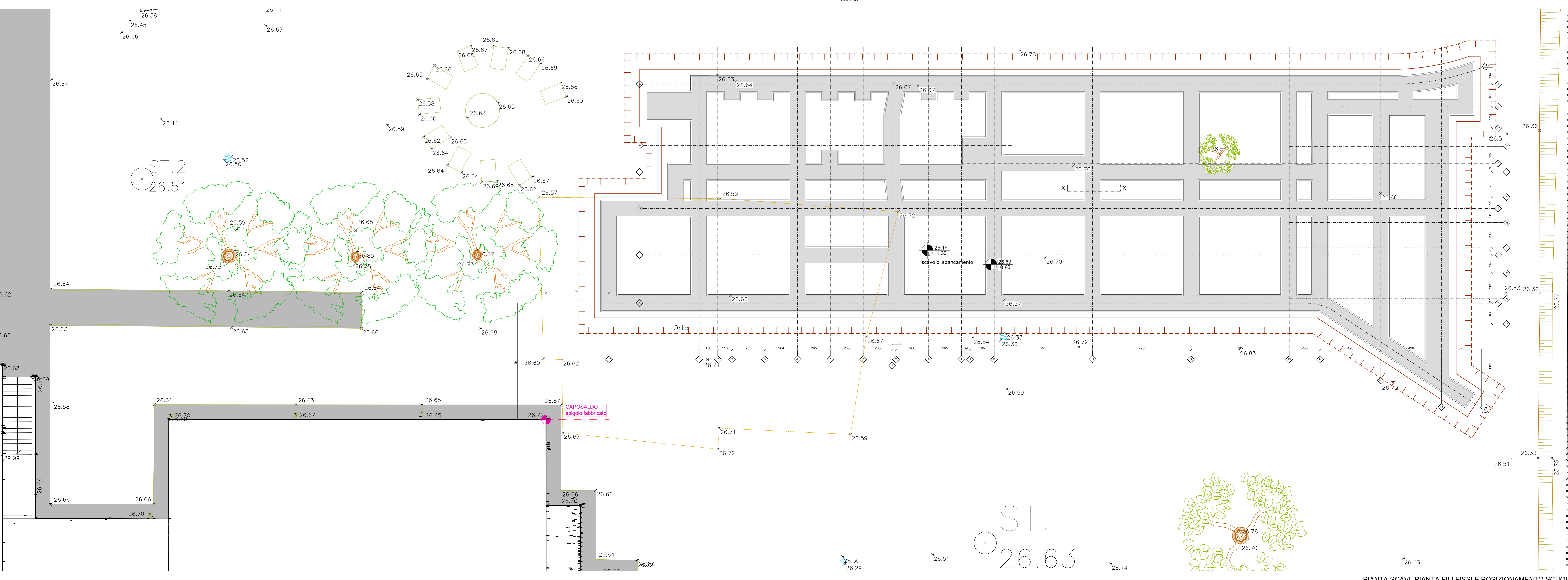
PIANTA SCAVI, PIANTE FILI FISSI E POSIZIONAMENTO SCUOLA Scala 1:100
