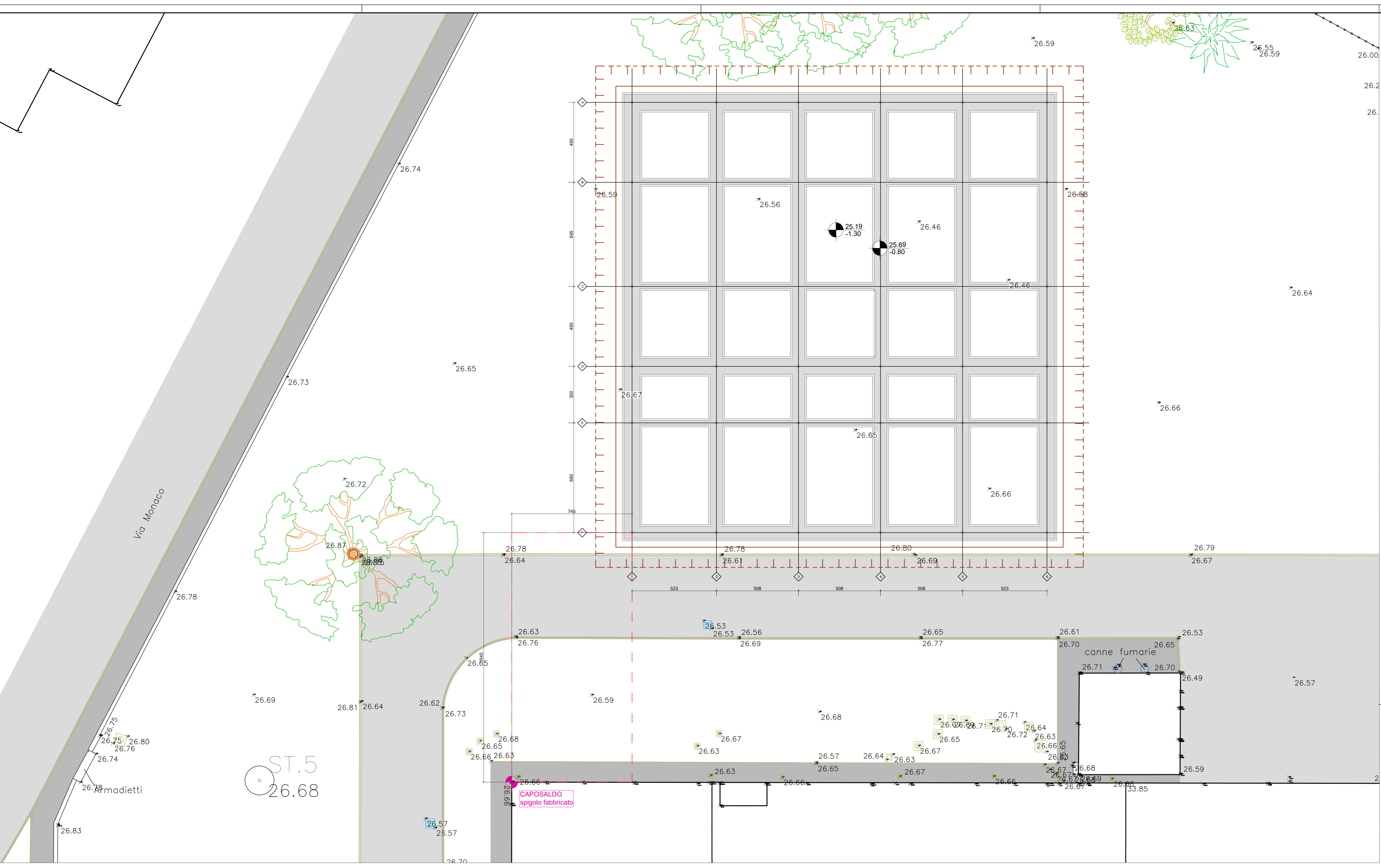
PIANTA SCAVI, PIANTE FILI FISSI E POSIZIONAMENTO PALESTRA Scala 1:100
