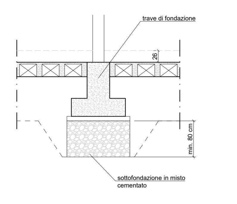
DETTAGLIO FONDAZIONE - SEZIONE X-X Scala 1:50
